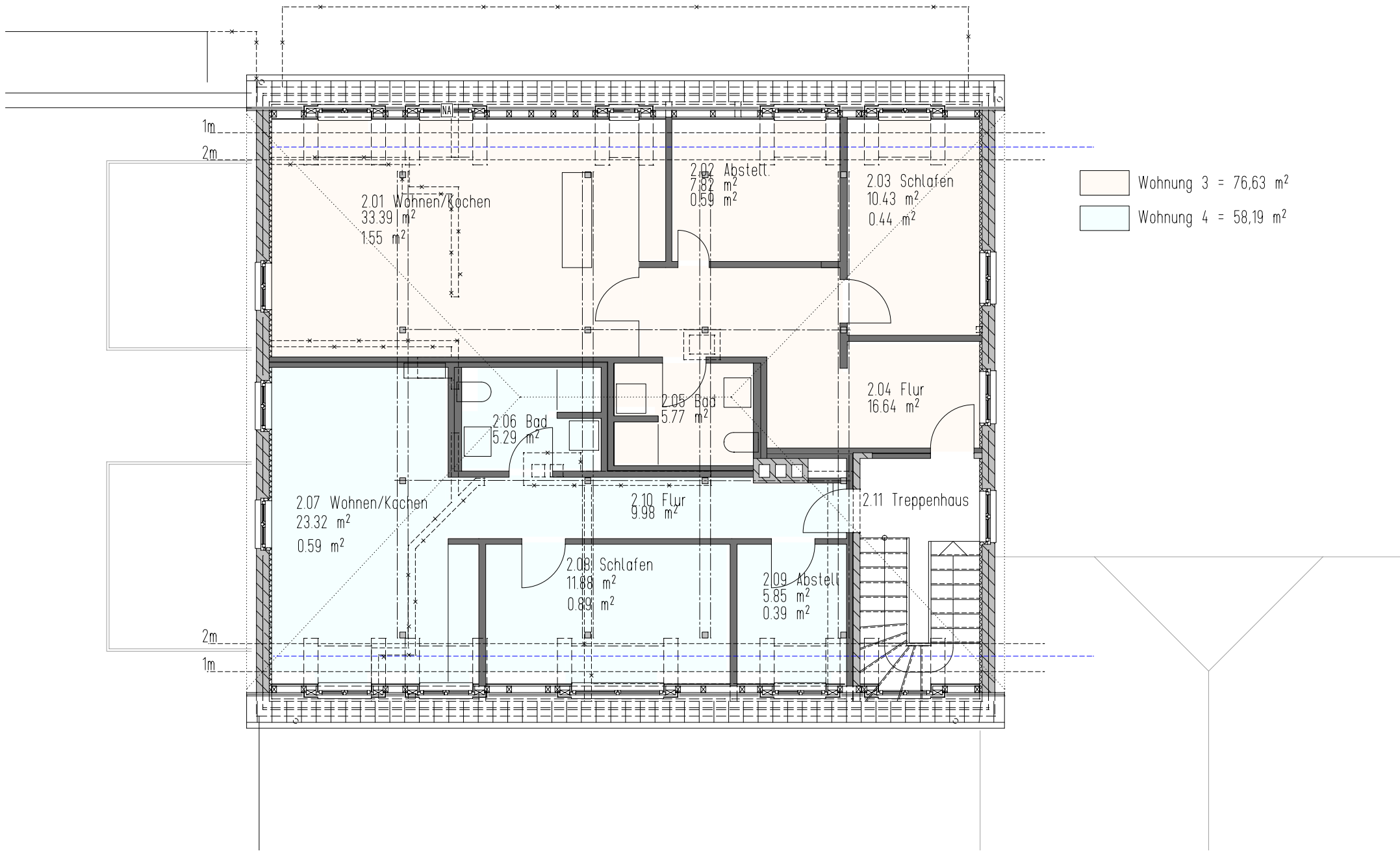
Bv 654 - Umnutzung mit Umbau eines Geschäftshauses in ein Ärztehaus mit Wohnungen / Hauptstr. 5 / 26340 Zetel Anlage zur Wohnflächenberechnung nach WoFIV
